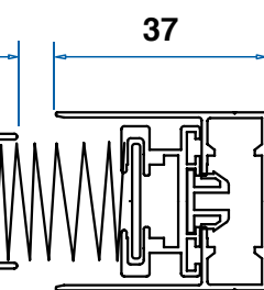
Profilo portarete
