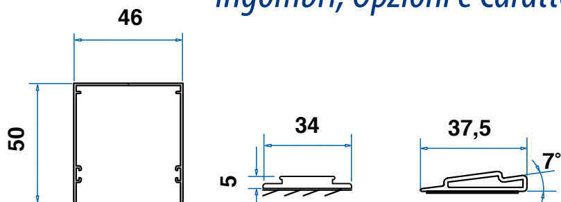
Guida superiore Maxxy
